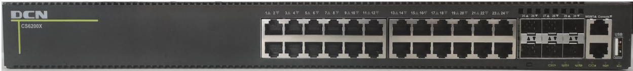
图 1-6 CS6200X-24T6X（-P）-EI 前面板
