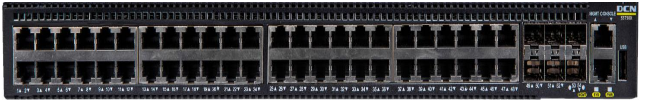
图 1-10 S5750X-48T6X（-P）-SI 前面板
