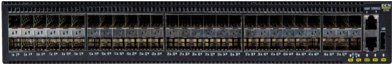
图 1-9 S5750X-48S6X-EI 前面板
