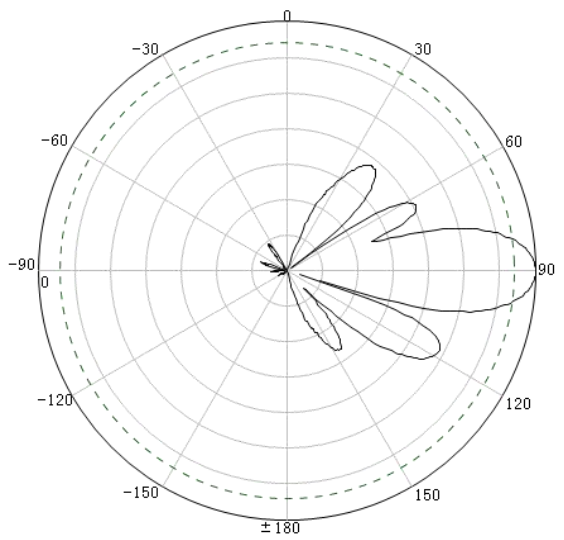
1 端口 E 面
