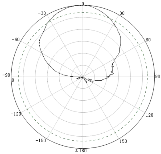
1 端口 H 面
