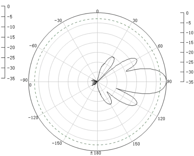
2 端口 E 面
