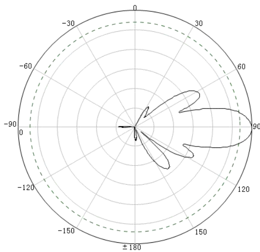
1 端口 E 面
