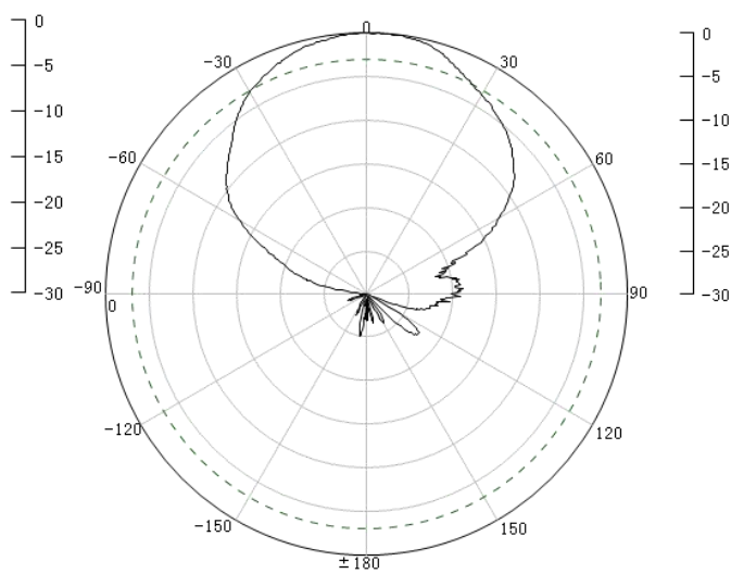
2 端口 H 面
