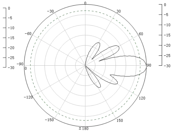
2 端口 E 面
