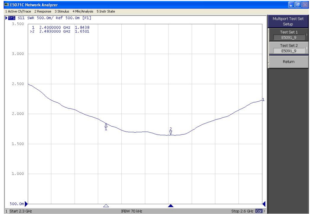
2 端口驻波图
