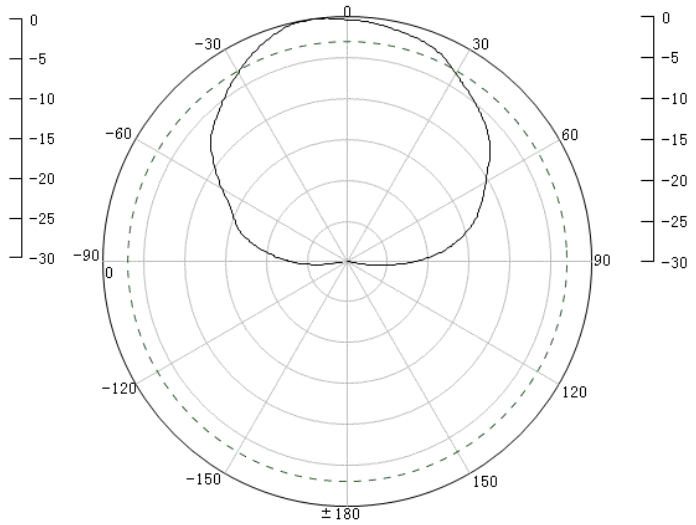
2 端口 H 面
