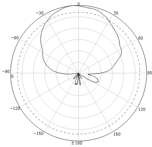
1 端口 H 面
