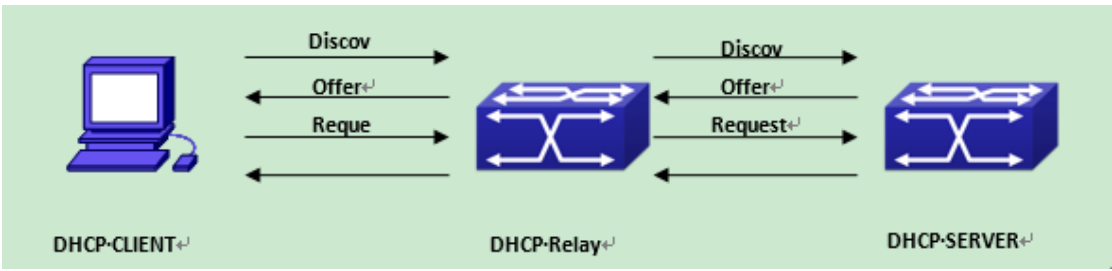
图 3-14 DHCP 中继
