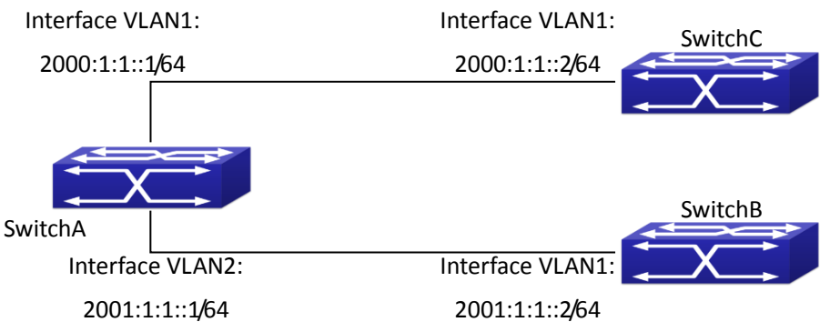
图 11-6 RIPng 案例
