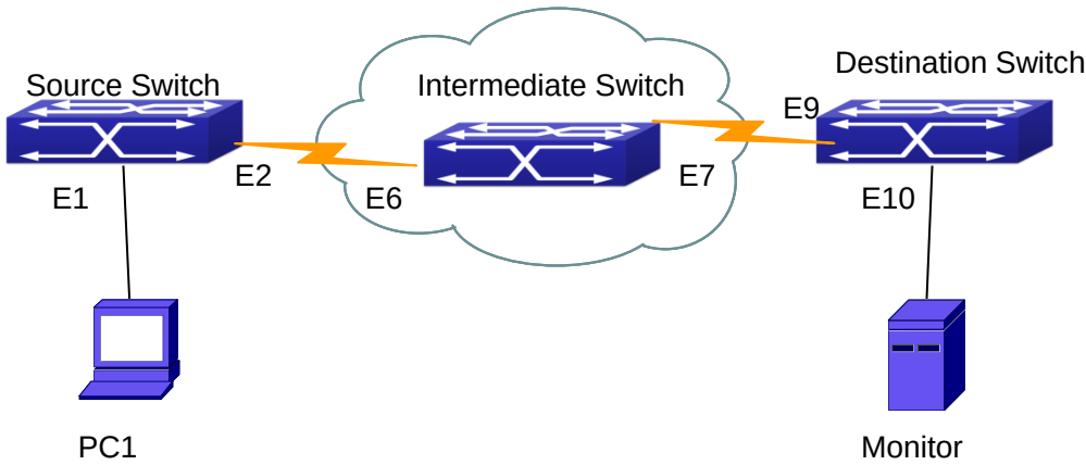
图 8-1 RSPAN 应用示意图
