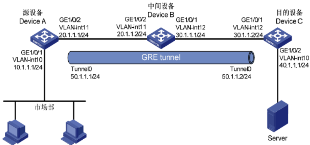
图 8-1 ERSPAN 应用示意图
