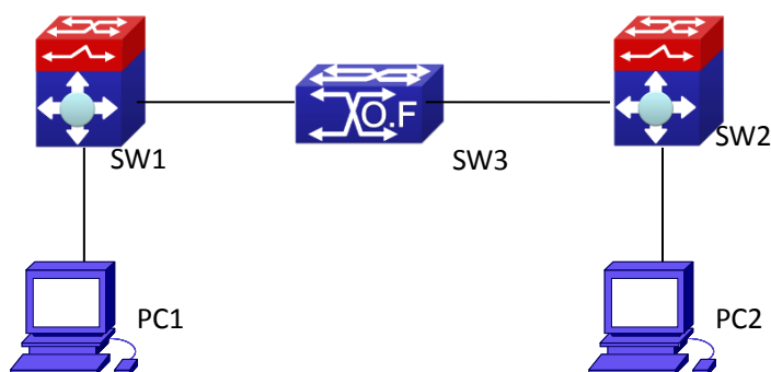
图 3-3 IPv6 隧道
