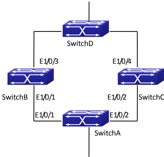
图 7-14 ULSM 典型配置案例
