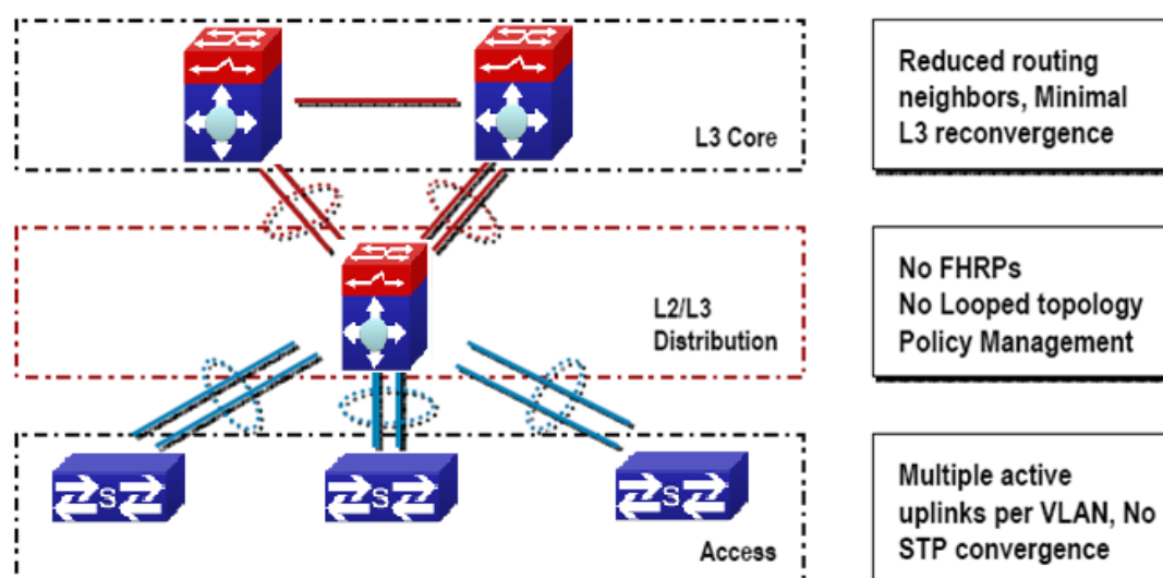
图 10-3 用虚拟化技术的企业网
