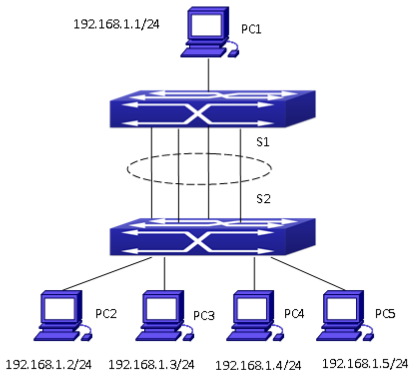
图 2-12 Load Balance 组网图
