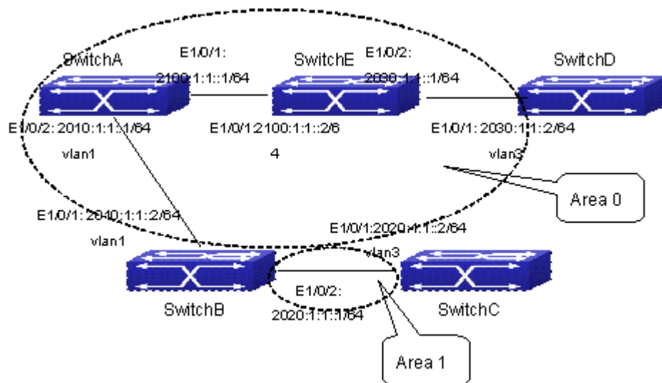
图 11-8 OSPFv3 自治系统网络拓扑示意图
