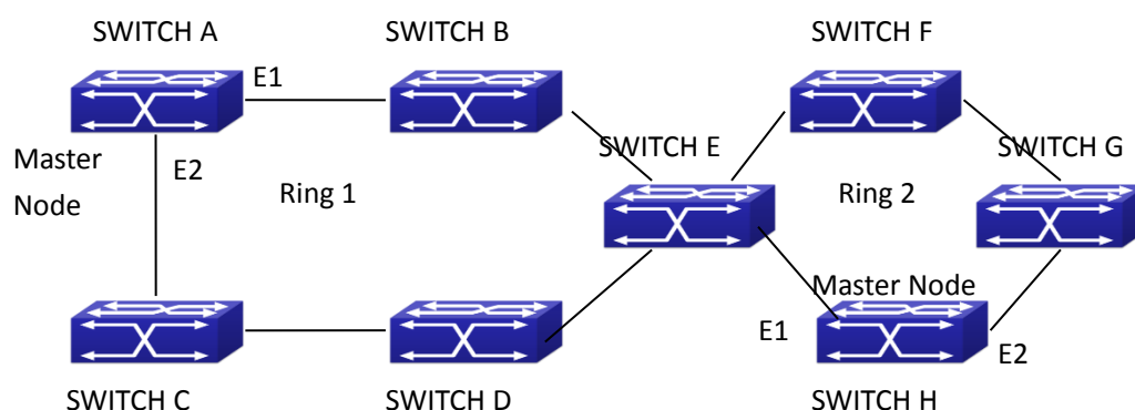
图 7-7 MRPP 示意图
