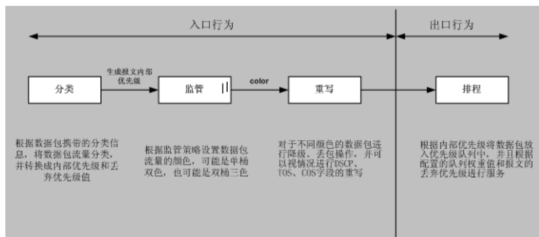
图 6-43 QoS 基本模型
