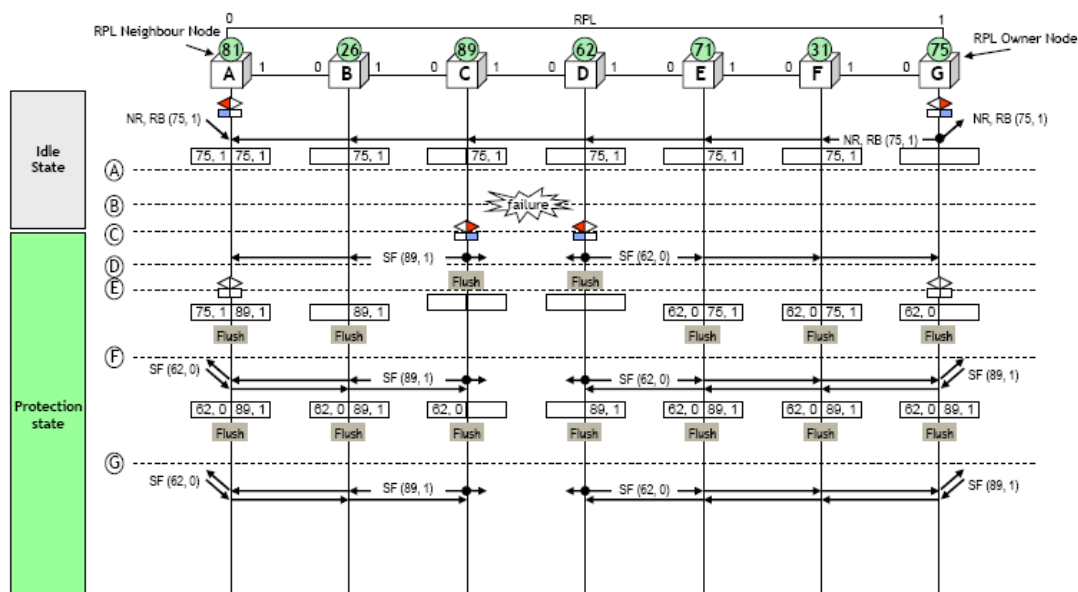
图 7-1 链路故障
