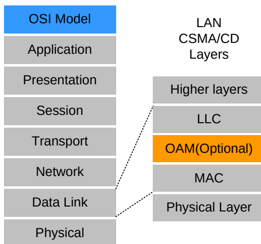
图 2-15 OAM 在 OSI 参考模型中的位置
