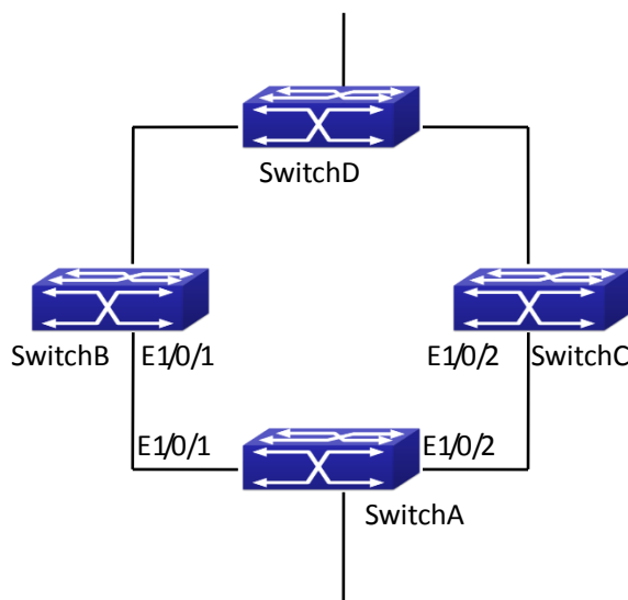
图 7-11 ULPP 典型配置案例 1
