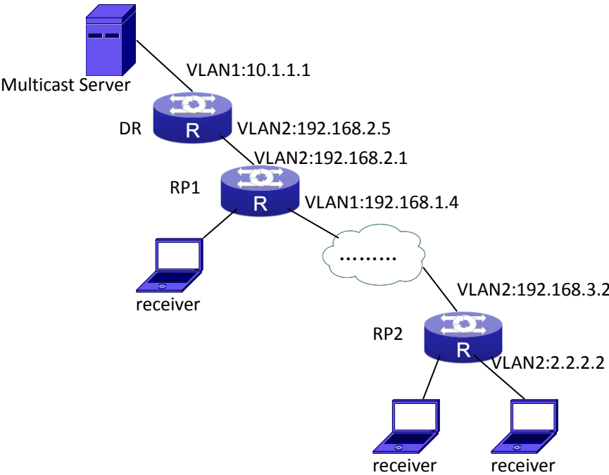
图 5-7 路由器 ANYCAST RP v4 功能
