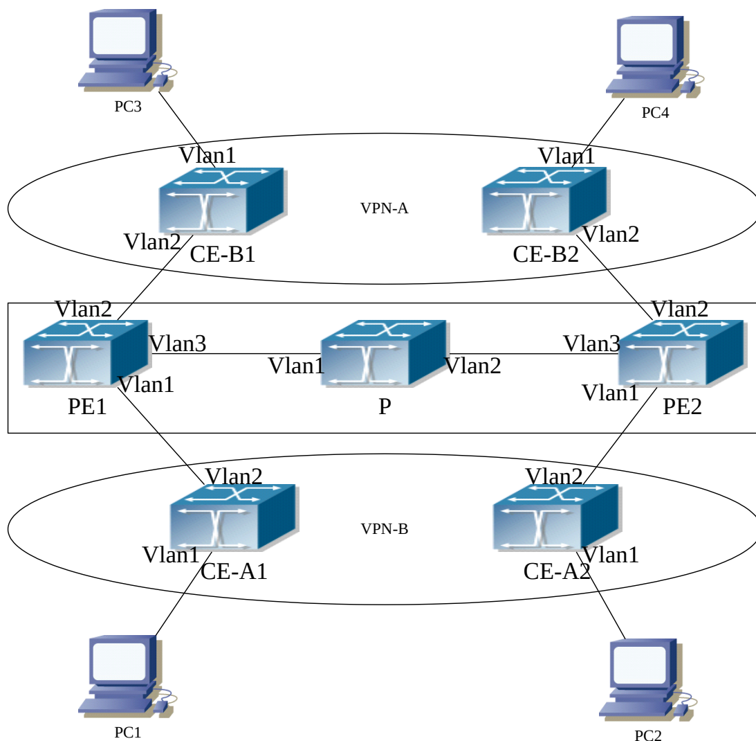
图 4-13 MPLS VPN 典型案例
