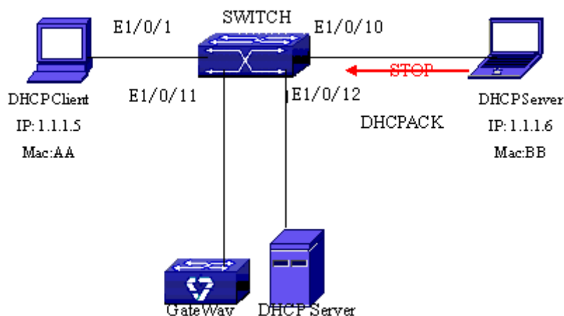
图 3-18 DHCP Snooping 防止非法 dhcp server 示意图
