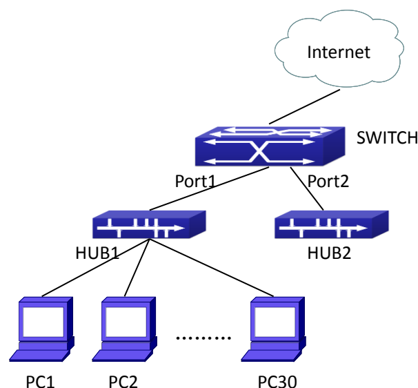
图 6-19 AM 功能典型配置案例
