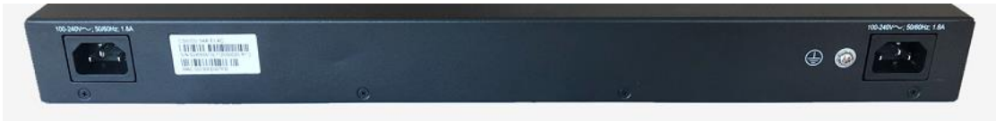
图 1-7 CS6200-54X-EI-XC 后面板
