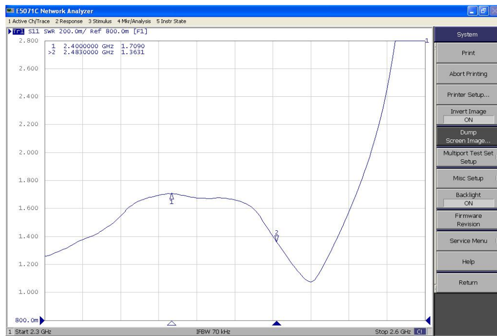
2 端口驻波图
