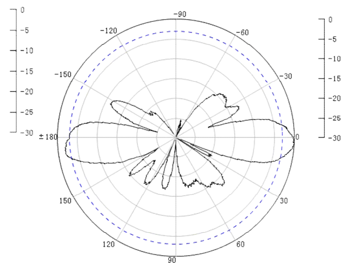
2 端口 E 面
