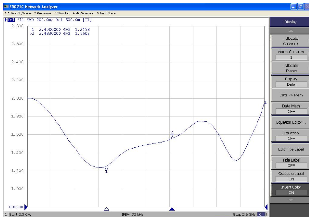
1 端口驻波图
