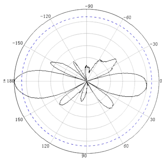
1 端口 H 面
