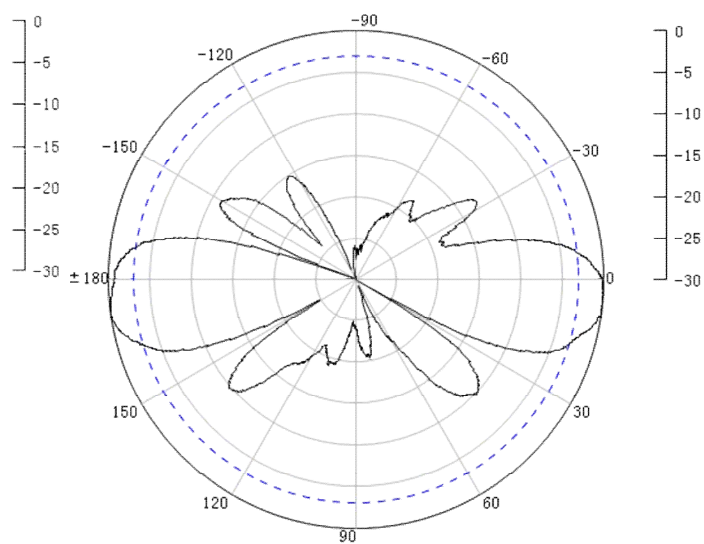
2 端口 E 面
