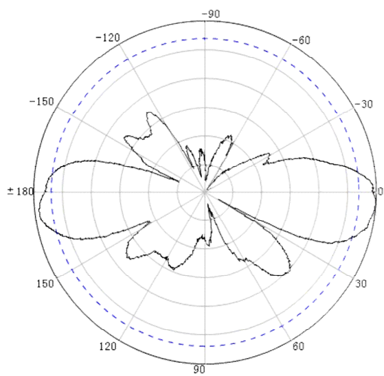
1 端口 E 面
