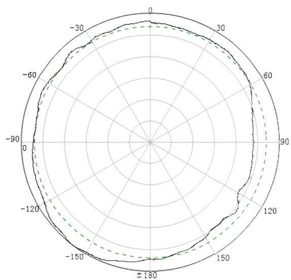
1 端口 H 面
