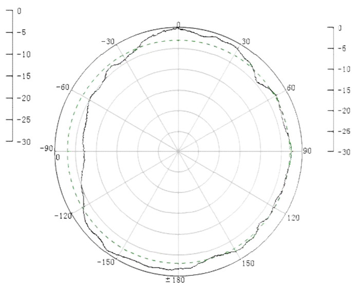
2 端口 H 面
