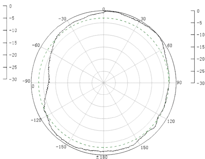
2 端口 H 面
