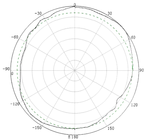
1 端口 H 面
